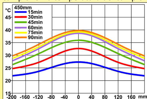
Temperatura dal centro ai bordi, dopo tempi diversi, per 450 mm di distanza tra il campione e il riscaldatore
