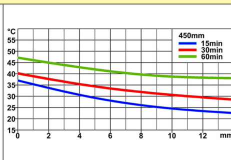
Penetrazione del calore all'interno del campione dopo diversi tempi di riscaldamento, a 450 mm di distanza tra il campione e il riscaldatore
