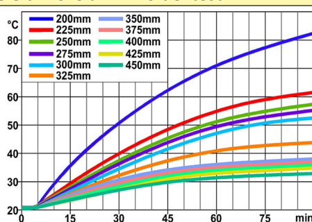
Temperatura media al centro del campione rispetto al tempo, a diverse distanze tra il campione e il riscaldatore.
